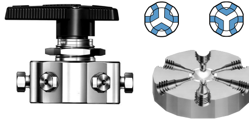
Vanne 6 voies
