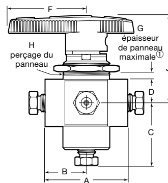
Vanne 5 voies
