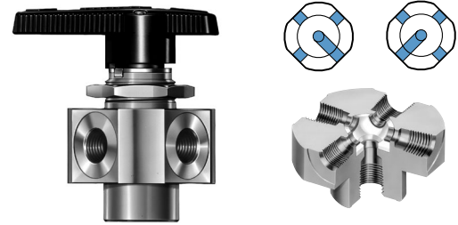
Vanne 5 voies
