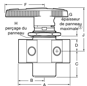
Vanne 7 voies
