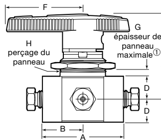
Vanne 4 voies
