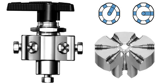
Vanne 7 voies
