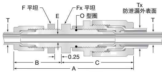
图中画出了卡套管。O 型圈为 Aflas®。
