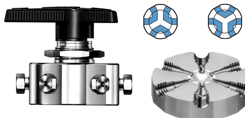
Vanne 6 voies
