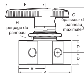
Vanne 6 voies
