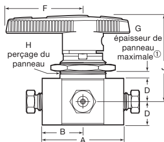
Vanne 4 voies
