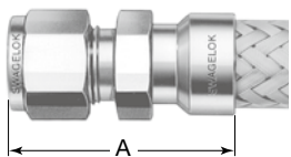
手動溶接型 (1インチ・サイズ超)
