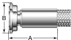
サニタリー用 DIN 11864-3 シリーズ A、Form A、 溝付きクランプ・フェルル①
