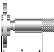
JIS 10K ラップ・ジョイント・フランジ
