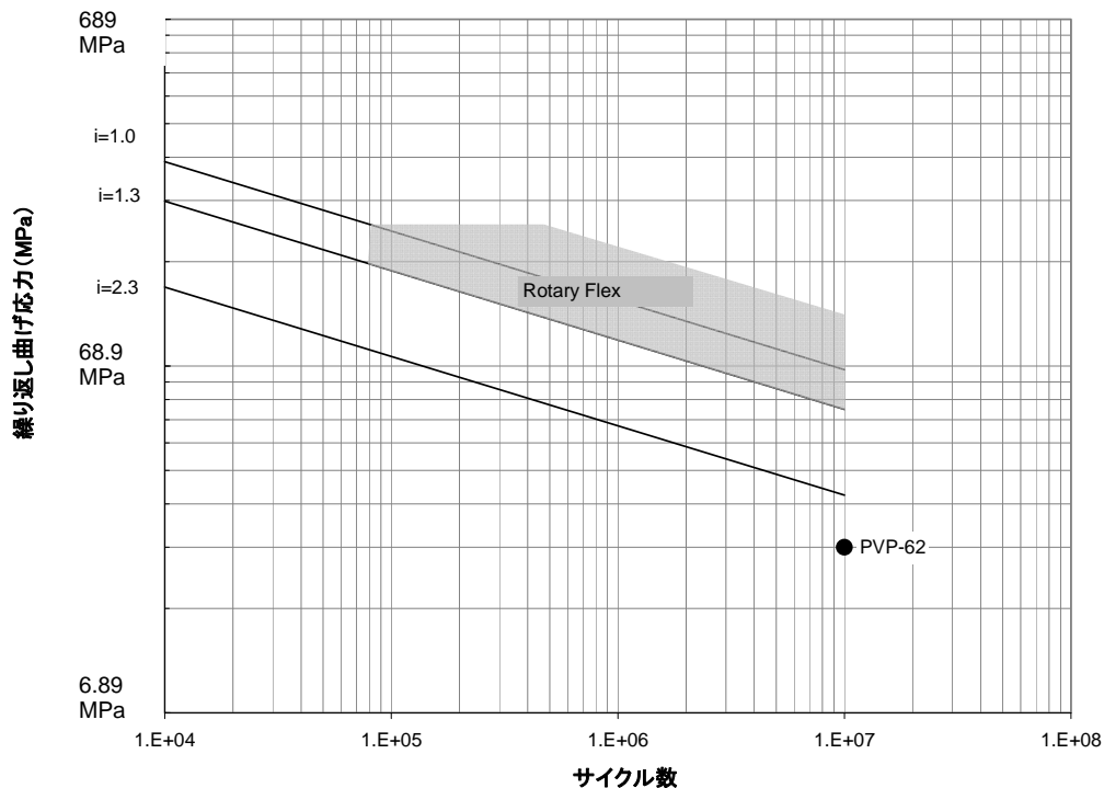
ステンレス鋼製 Swagelok ミディアム・プレッシャー・チューブ継手の回転曲げ試験
