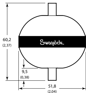
Модели HFS4A и HFS4B
